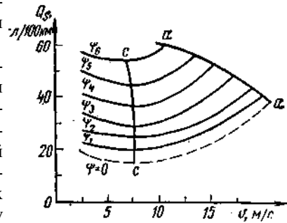
Рис. 4.7. Экономическая характеристика автомобиля
