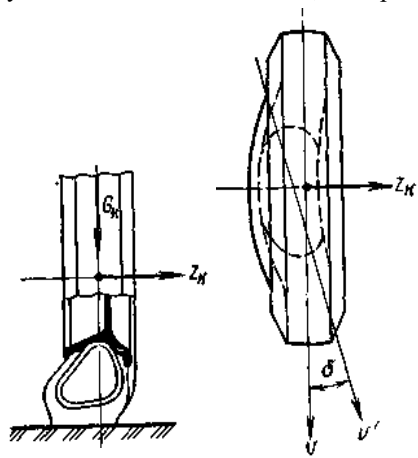
Рис. 3.3. Схема бокового увода шины
