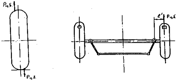
Рис. 6.5. Влияние несбалансированности колеса на его качение
