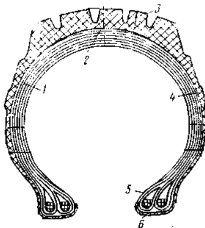
Рис. 3.1. Конструктивные элементы пневмошины:
