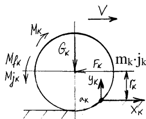
Рис. 3.5. Движение колеса по деформирующейся поверхности
