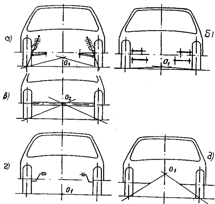
Центры крена кузова автомобиля
