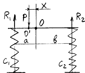
Рис. 7.2. Колебательная система с 4 упругими элементами
