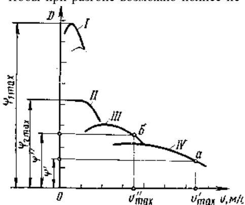
Рис. 4.3. Динамические характеристики автомобиля
