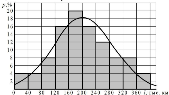
Рисунок 3 – Распределение ресурса двигателей КАМАЗ-ЕВРО
