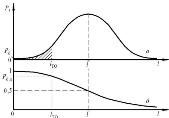
Рисунок 5— Распределение наработки на отказ l ( a ) и вероятность безотказной работы P_0 ( b )
