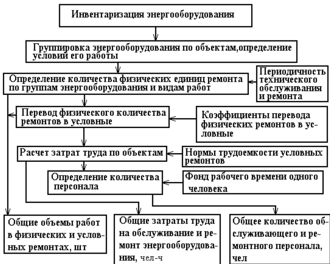
Рисунок 1 - Схема расчета объемов и стоимостей работ по обслуживанию и ремонту энергооборудования в хозяйстве
