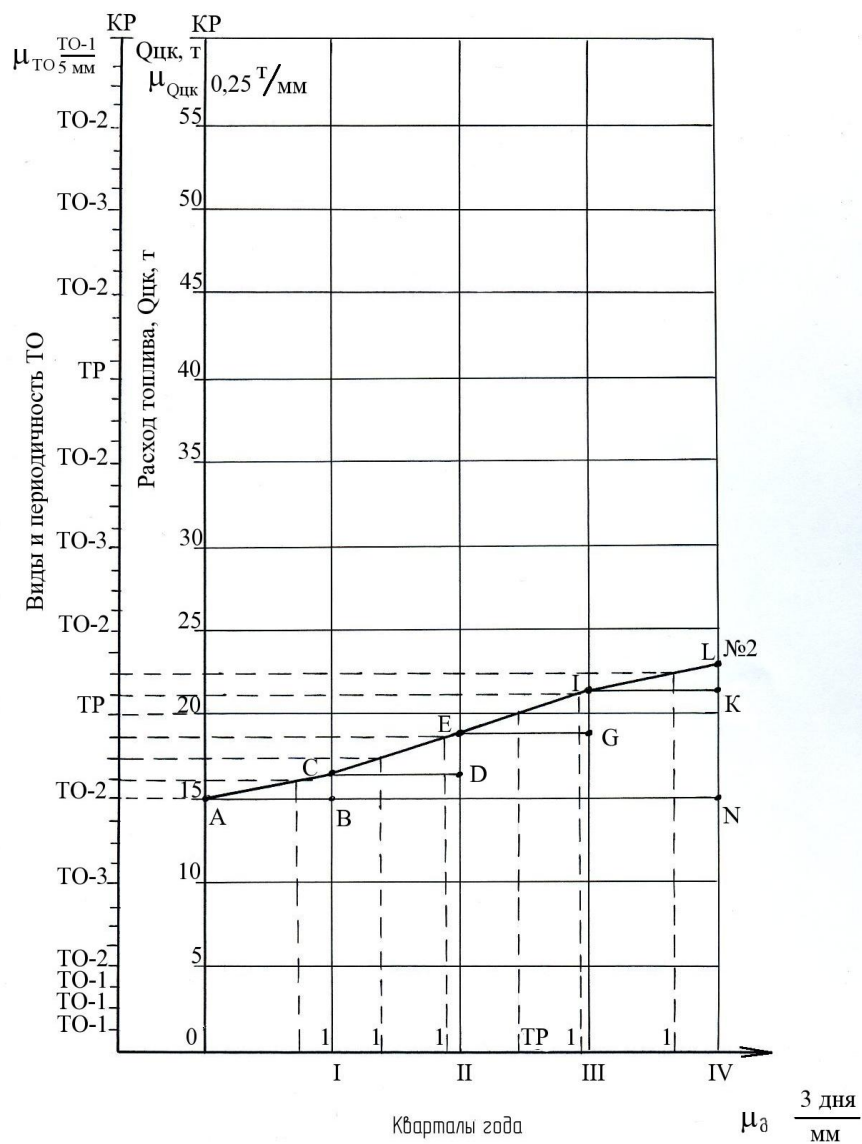
Рисунок 2.1 - Графический способ планирования ТО трактора ВТ-100Д
